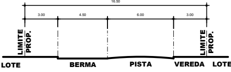
SECCION A-A CALLE 2 ESCALA 1/250
