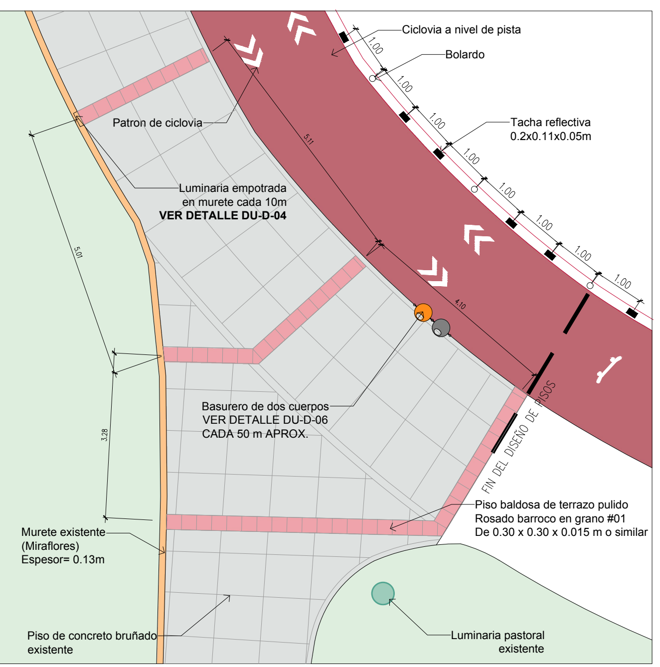
PLANTA DETALLE INICIO DEL PARQUE DOMODOSSOLA - MIRAFLORES ESCALA: 1:75
