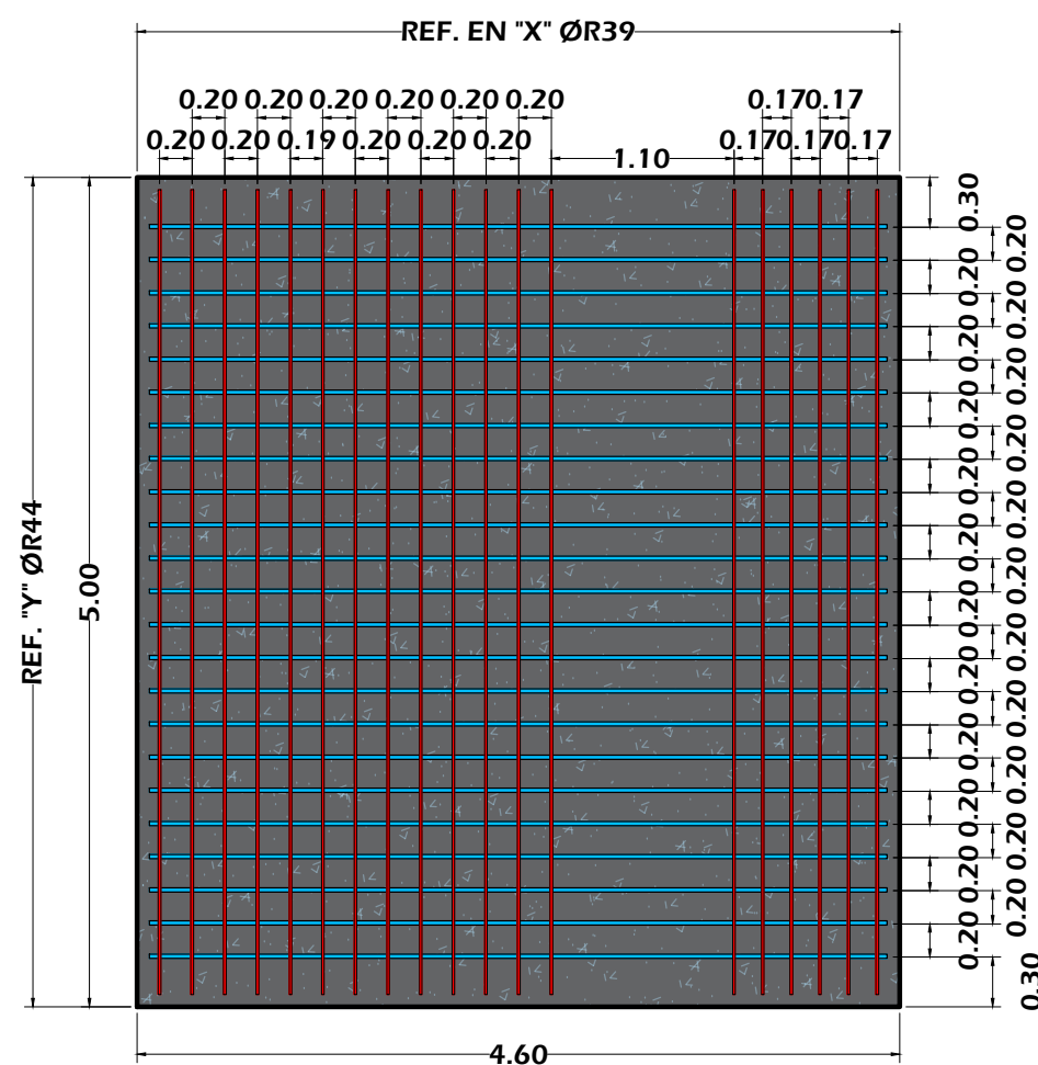
DISTRIBUCIÓN DEL REFUERZO SUPERIOR EN ZAPATA DE ESTRIBO (vista en planta) ESCALA: 1/50
