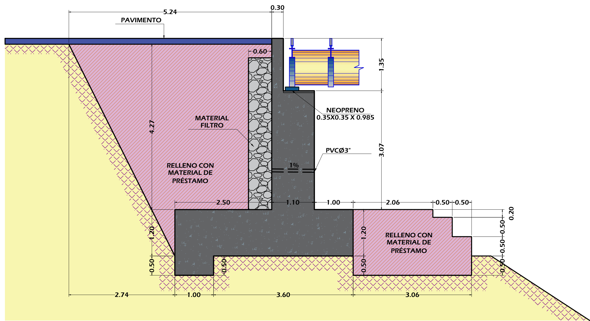
DIMENSIONES DE ESTRIBO ESCALA: 1/50
