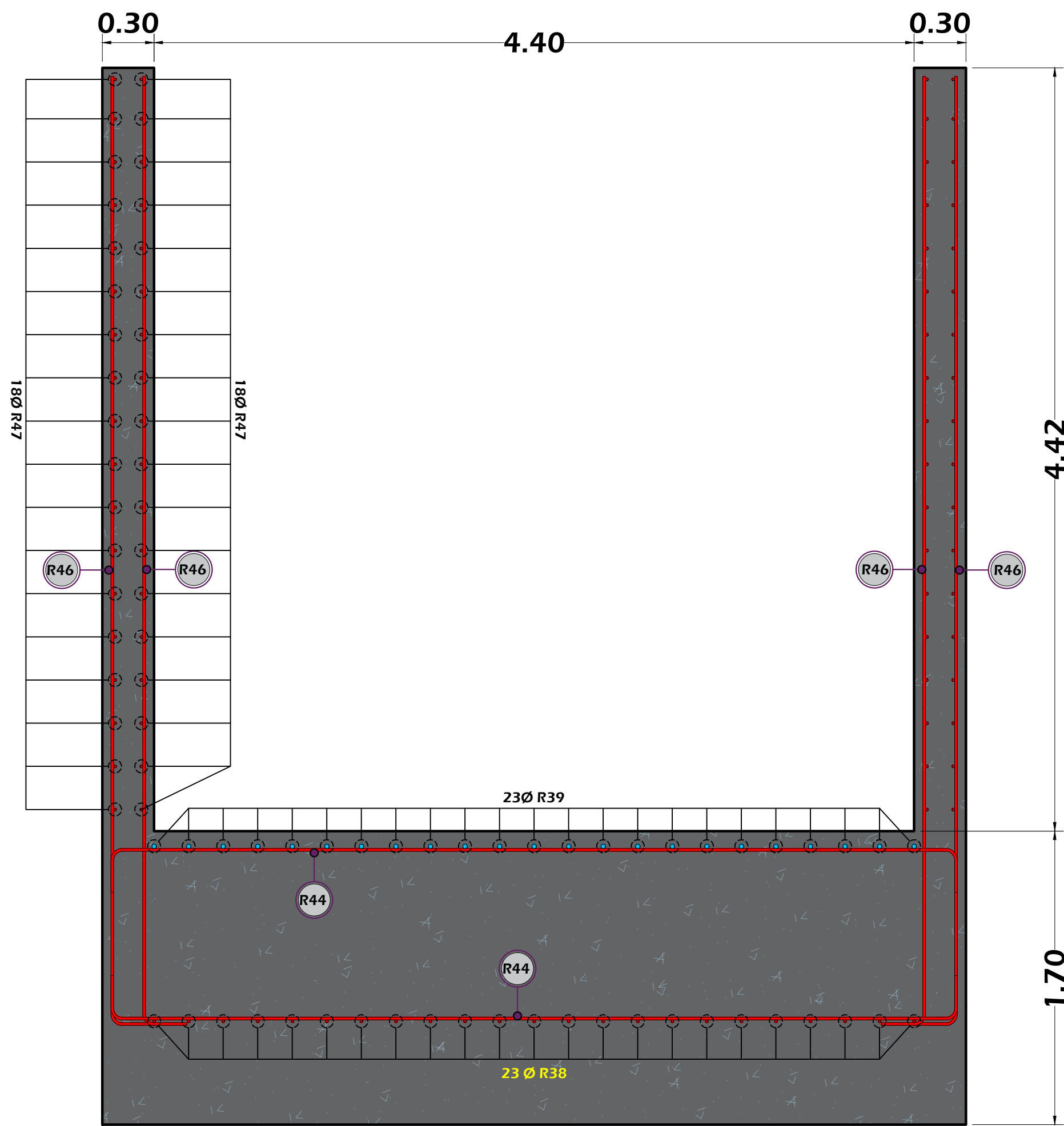
ACERO DE REFUERZO EN ALAS DE ESTRIBO SEGÚN CORTE h'-h' ESCALA: 1/25
