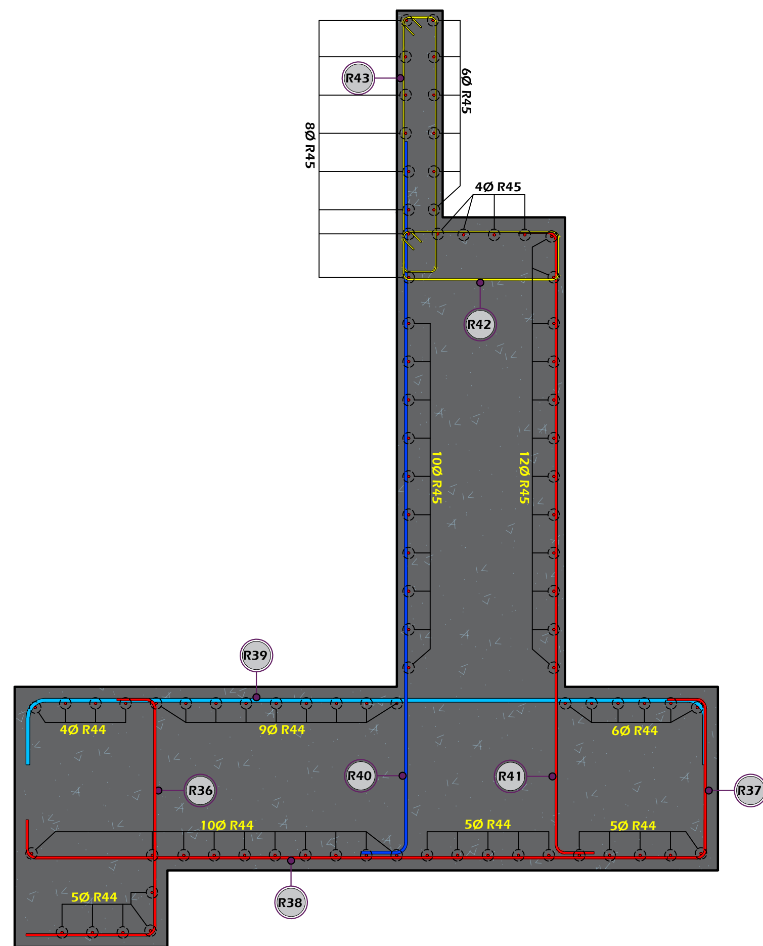
ACERO DE REFUERZO EN ESTRIBO SEGÚN CORTE g'-g' ESCALA: 1/25
