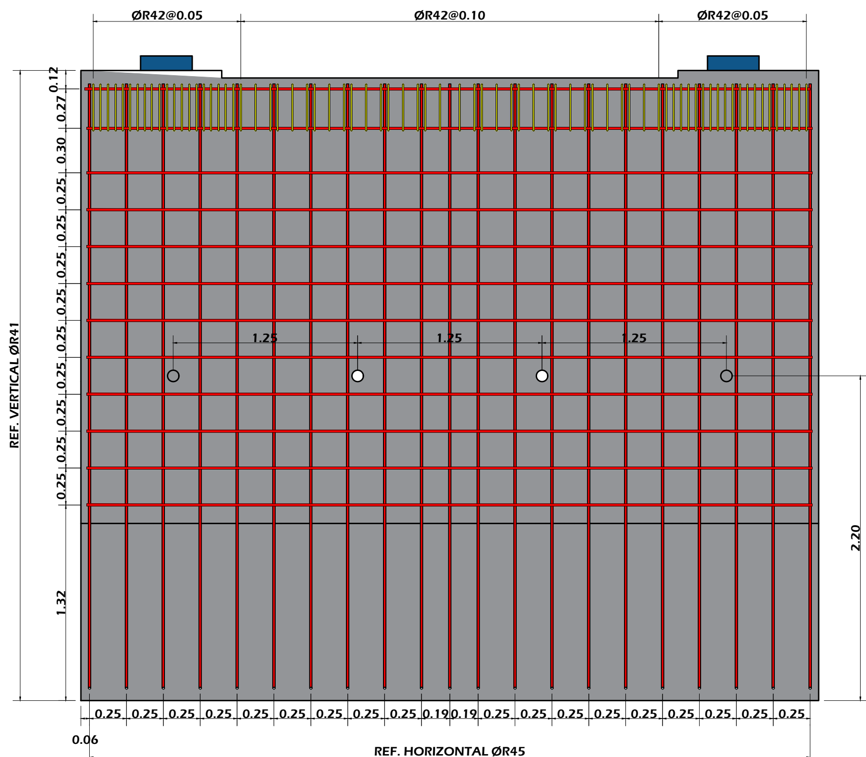
DISTRIBUCIÓN DE REFUERZOS EN PNATALLA CARA EXPUESTA ESCALA: 1/25
