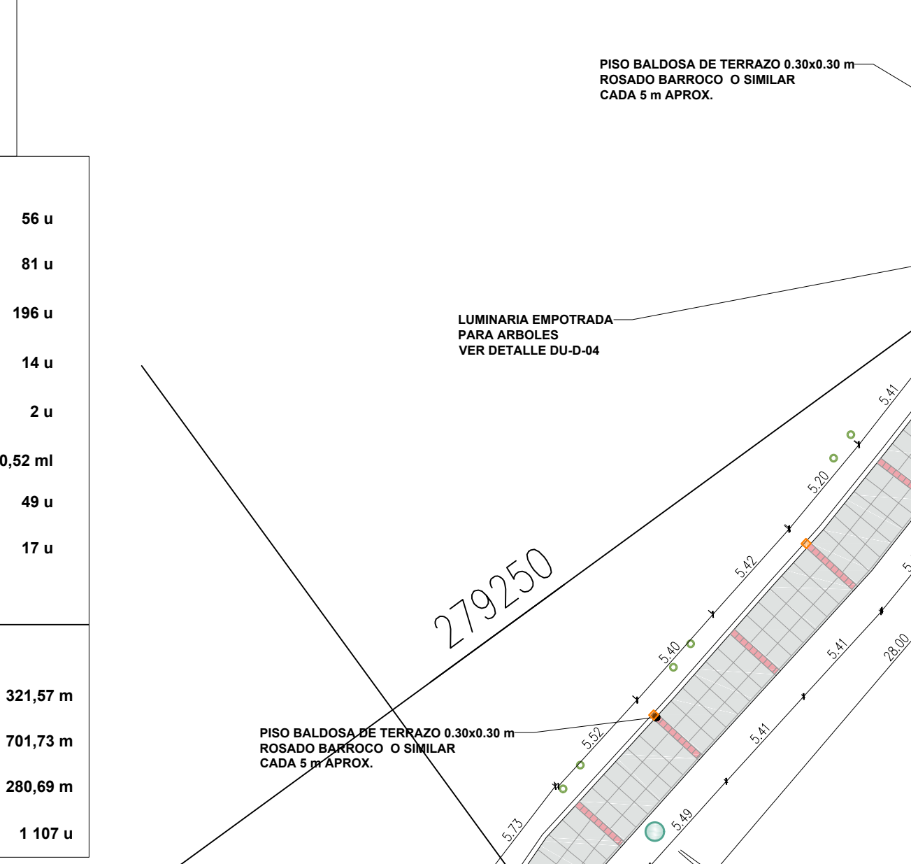
PLANTA DETALLE DE LUMINARIA EN MURETE Y ARBOLES - MIRAFLORES (PARQUE DOMODOSSOLA) ESCALA: 1:50
