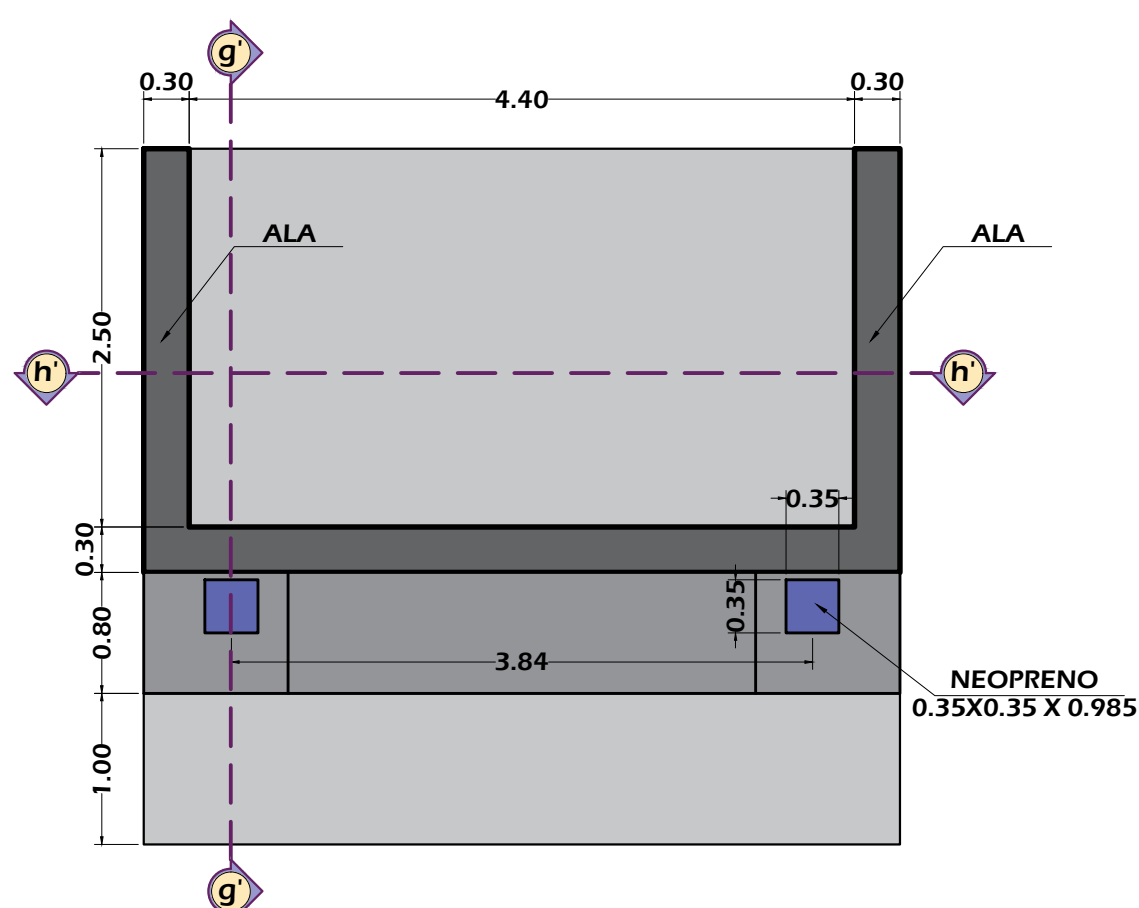
DIMENSIONES DE ESTRIBO (VISTA EN PLANTA) ESCALA: 1/50
