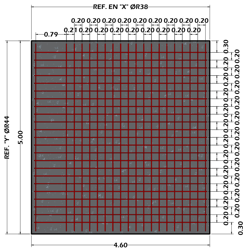
DISTRIBUCIÓN DEL REFUERZO INFERIOR EN ZAPATA DE ESTRIBO (vista en planta) ESCALA: 1/50
