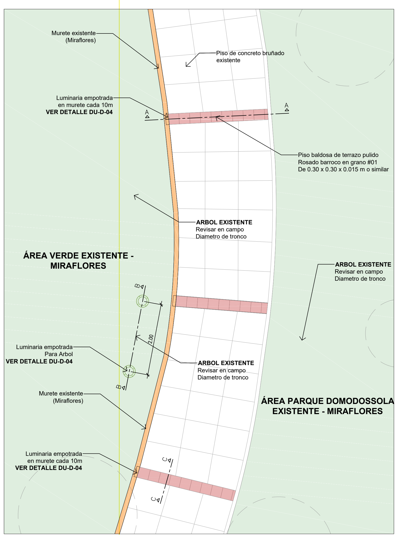
PLANTA DETALLE DE LUMINARIA EN MURETE Y ARBOLES - MIRAFLORES (PARQUE DOMODOSSOLA) ESCALA: 1:50
