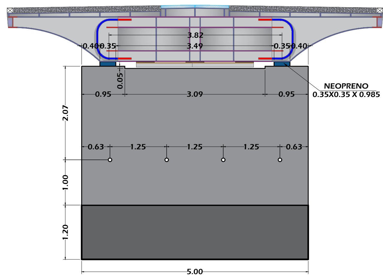
DIMENSIONES DE ESTRIBO (VISTA FRONTAL) ESCALA: 1/50
