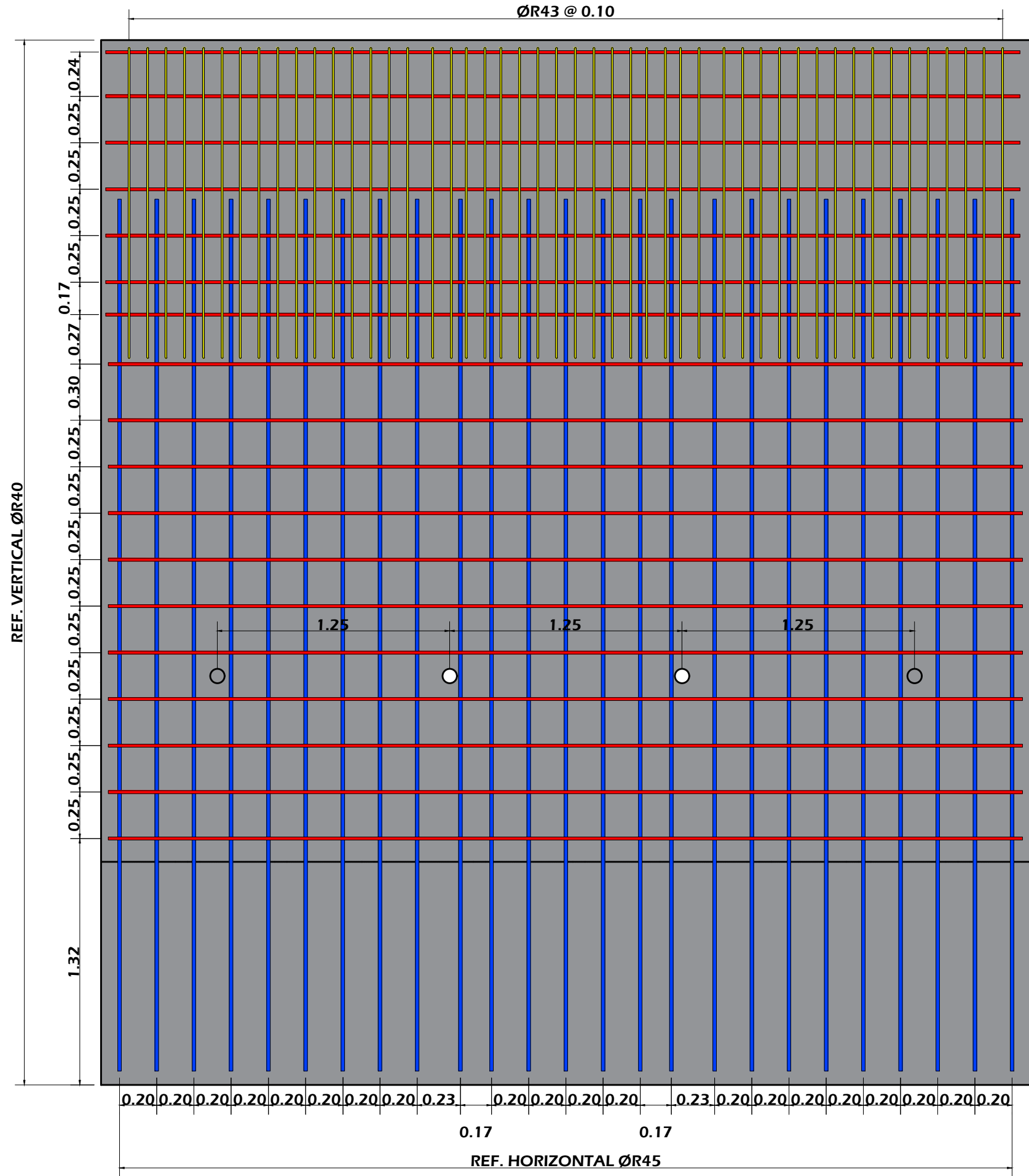
DISTRIBUCIÓN DE REFUERZOS EN PNATALLA CARA QUE DA HACIA EL RELLENO ESCALA: 1/25
