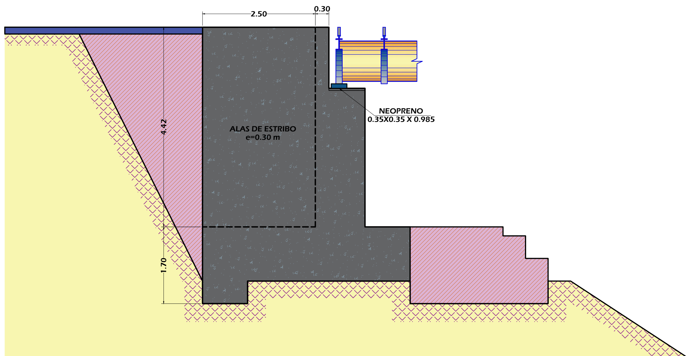
VISTA LATERAL DE ALAS DE ESTRIBO ESCALA: 1/50
