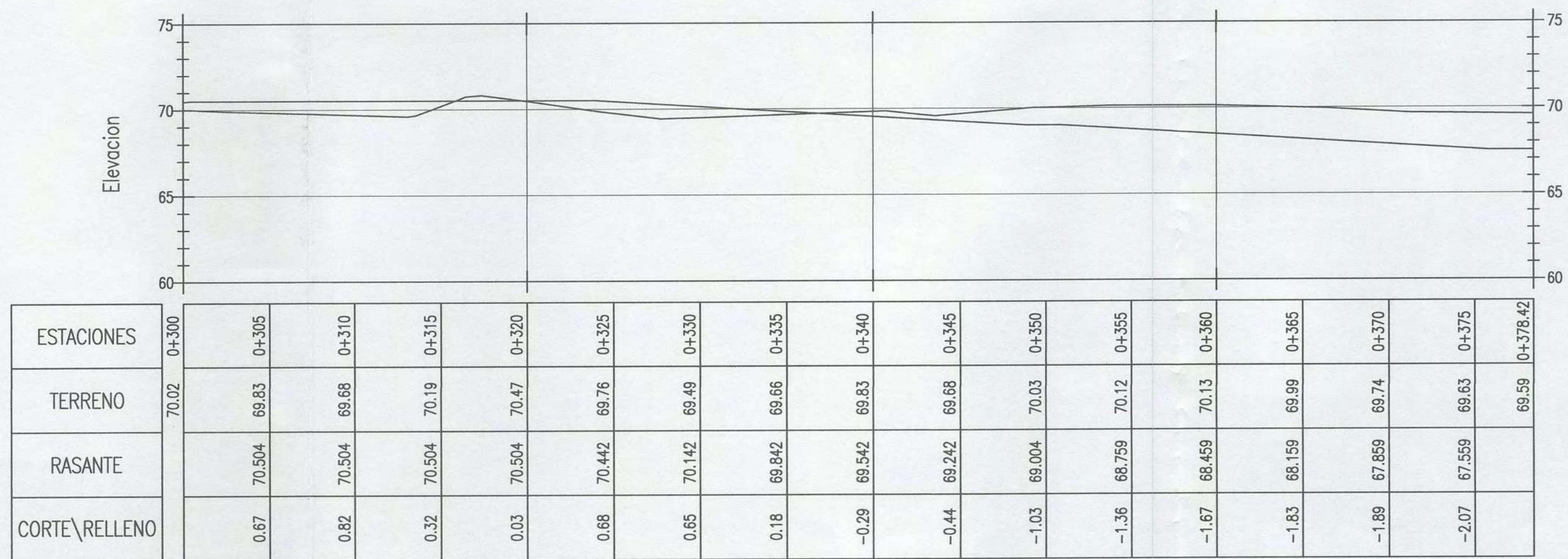
PERFIL DE EJE: EJE CAMINO PEATONAL 5
