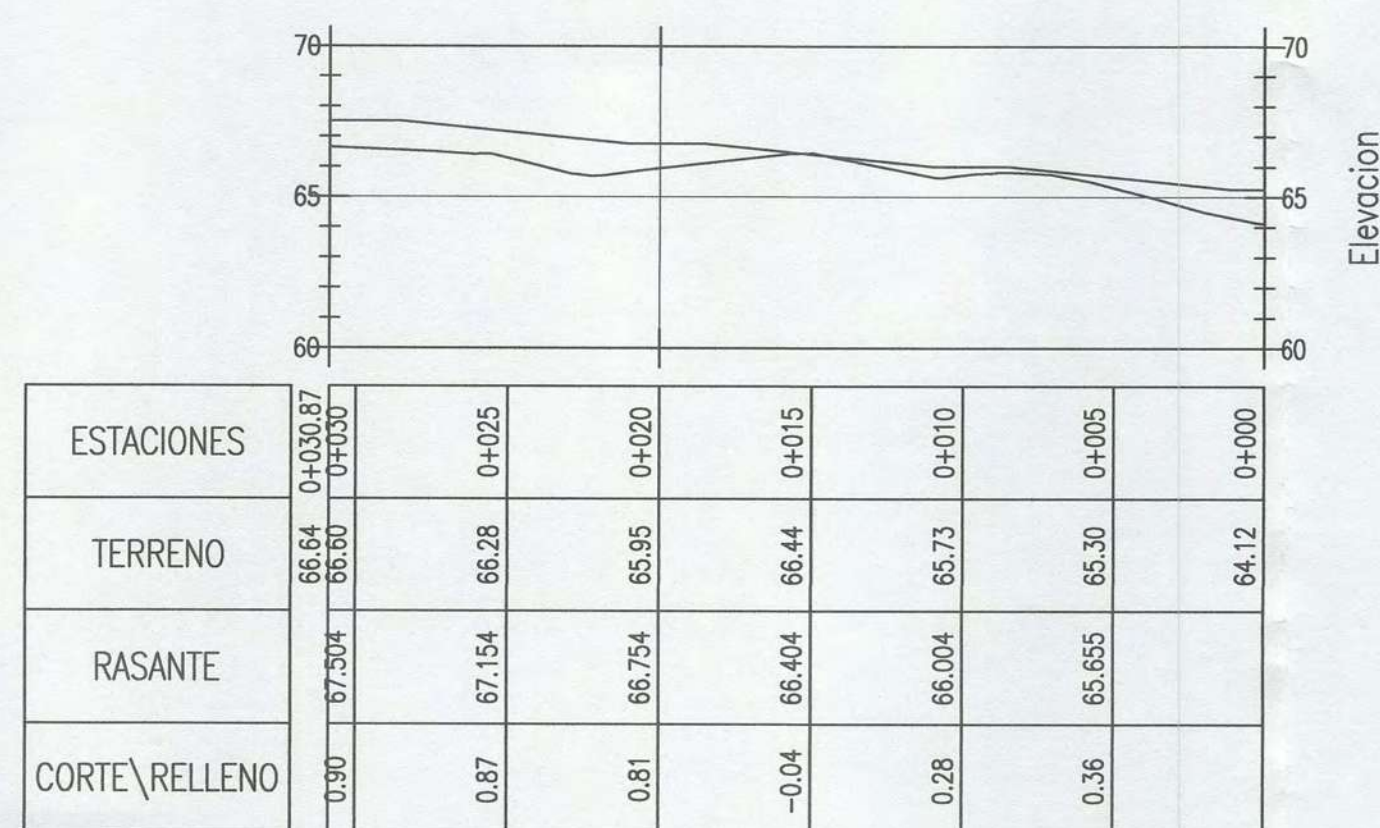
PERFIL DE EJE: EJE CAMINO PEATONAL 3
