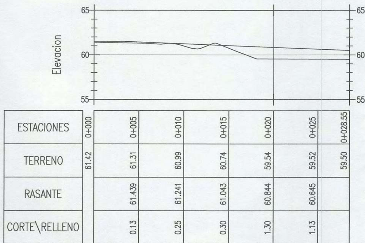
PERFIL DE EJE: EJE CAMINO PEATONAL 4
