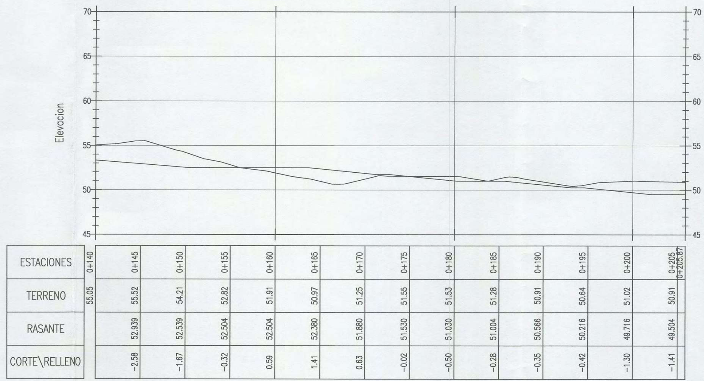
PERFIL DE EJE: EJE CAMINO PEATONAL 1
