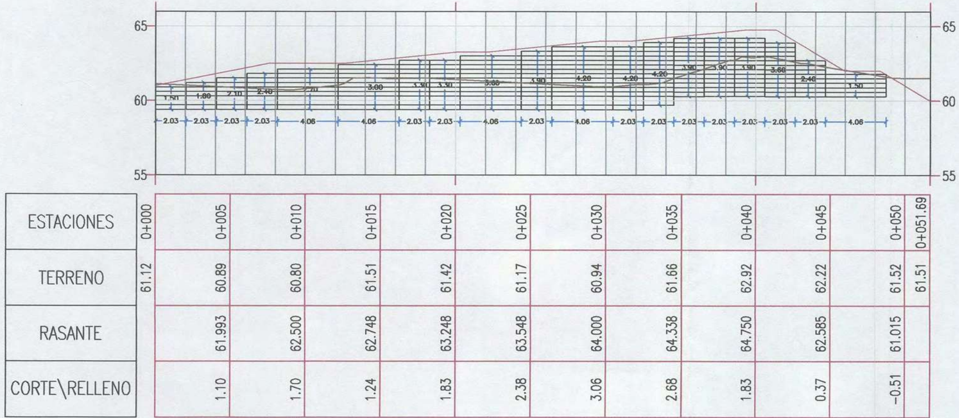
PERFIL DE EJE: EJE MURO 1
