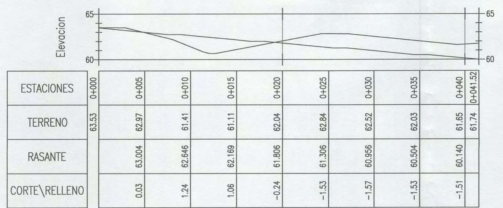
PERFIL DE EJE: EJE CAMINO PEATONAL 11
