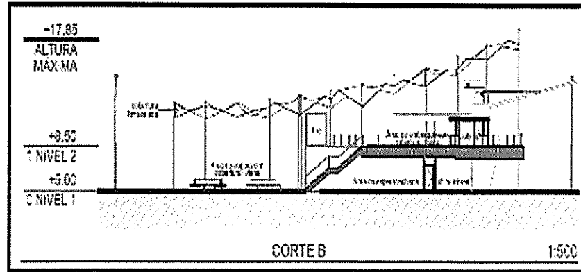
Gráfico N° 09 Plano de corte del Paradero Playa Redondo
