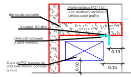
CORTE D-D Esc. 1/10
