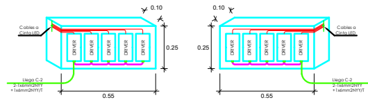
CAJA DE PASE F*G* DE 550X250X100MM CON TAPA HERMÉTICA Y SEGURO + LLAVE Esc. 1/10
