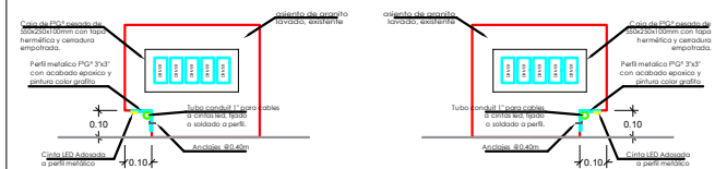
DETALLE 1 Esc. 1/10
